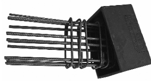
Typ/Type TSB-T Schall-Isobox/Boîte insonorisante Füllkörper/Remplissage Armierungskorb/Corbeille d'armature
