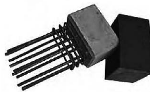
Typ/Type TSB-BT Schall-Isobox/Boîte insonorisante Füllkörper/Remplissage Beton-Tragelement/Élément porteur
