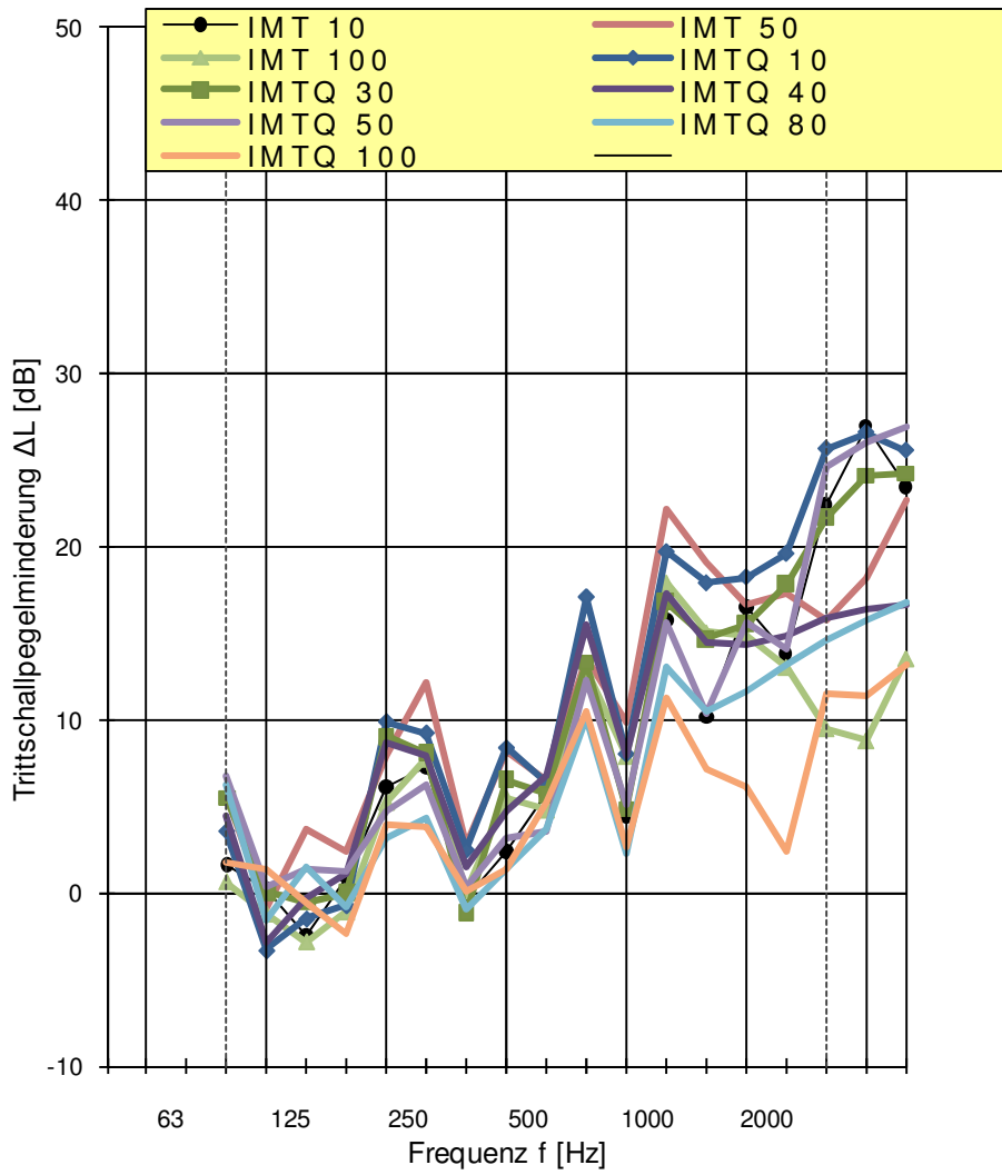
Diagramm 2: Frequenzverlauf der Trittschallpegelminderung \Delta L gegenüber dem durchbetonierten Anschluss
