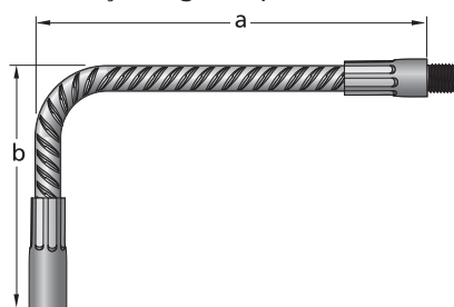
ANMUB Anschlussstab gebogen mit Muffe Barre de raccord à manchon avec façonnage simple
