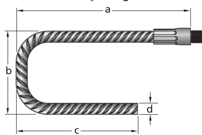
ANBB Anschlussstab 2 x gebogen Barre de raccord avec double façonnage
