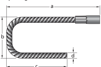
MUBB Muffenstab 2 x gebogen Barre à manchon avec double façonnage
