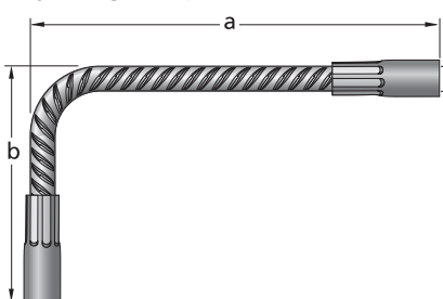
DMUB Doppelmuffenstab gebogen Barre à 2 manchons avec façonnage simple
