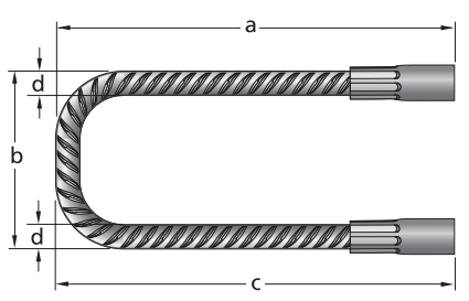
DMUBB Muffenbügel Etrier avec 2 manchons
