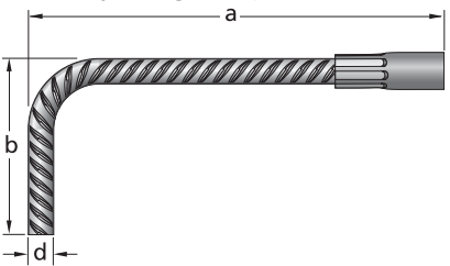
MUB Muffenstab gebogen Barre à manchon avec façonnage simple
