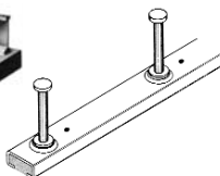
Ankerschiene JXA Rails d'ancrage JXA
