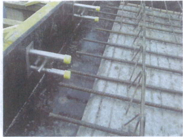
Bild 4. Einige Decken der Tiefgaragen werden unter zusätzlicher Verwendung vorgefertigter Filigrandecken gebaut; die gedrungene Bauweise der JORDAHL®-Doppelschubdorne ermöglicht auch hier einen unproblematischen Einbau
